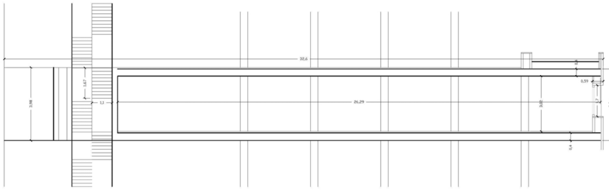
SECCIÓN A-A'
