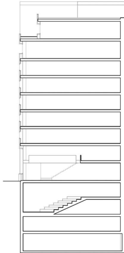
SECCIÓN GRAN VÍA
